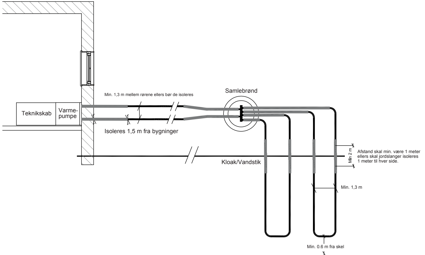
Plan for slangeudlægning.
